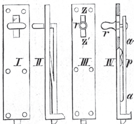
Obr. 33: Dvě varianty zapuštěné zástrčky (převzato z A. O. F. Večeř, o. c. v pozn. 12, s. 37, obr. 88).
