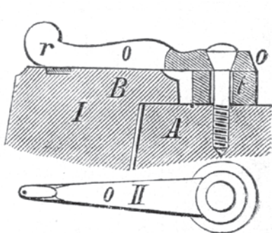
Obr. 24: a – vlevo: Večeř má nejucelenější přehled obrtlíků určených pro zavírání jednoho křídla okna od nejjednodušších připevněných vrutem či zanáťovanými do plechu; b – vpravo: v dokonalejších případech okenní lištu chránil drát či plíšek s ozubem (převzato z A. O. F. Večeř, o. c. v pozn. 12, s. 34–35, obr. 76 a 77).
