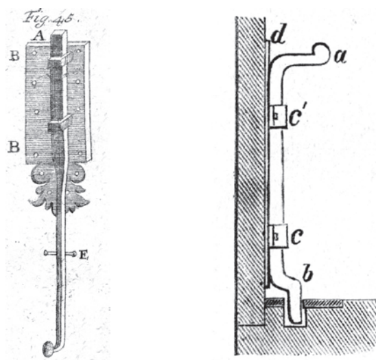
Obr. 32: Nejjednodušší typ nasazené zástrčky u dvoukřídlých dveří, kde byly obvykle párově: a – nahoře (převzato z H-L. Duhamel du Monceau, o. c. v pozn. 4, tab. 13, obr. 45) a b – dole (převzato z A. O. F. Večeř, o. c. v pozn. 12, s. 37, č. 85); c – mezi tyto zástrčky náleží i nejjednodušší utilitární typy – Žatec (okres Louny) čp. 102.
