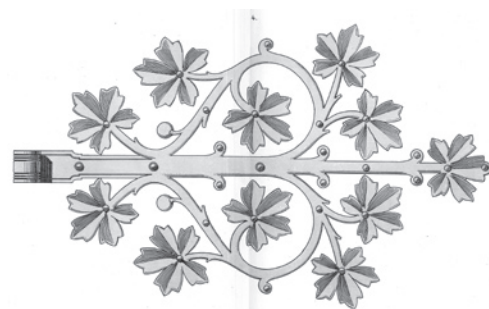
Obr. 8: Postupem vývoje se tvary předloze dále vzdalovaly. Odlišnosti od původního tvaru jsou snad nejmarkantnější u neogotických kování. V tomto případě dobová literatura nazývá křížovými závěsy i velmi bohaté neogotické závěsy vesměs s vegetabilním dekorem. Podobných příkladů je více (převzato z J. Storck – G. Gugitz – F. Paulik, o. c. v pozn. 10, sv. 2., tab. 6, 7).
