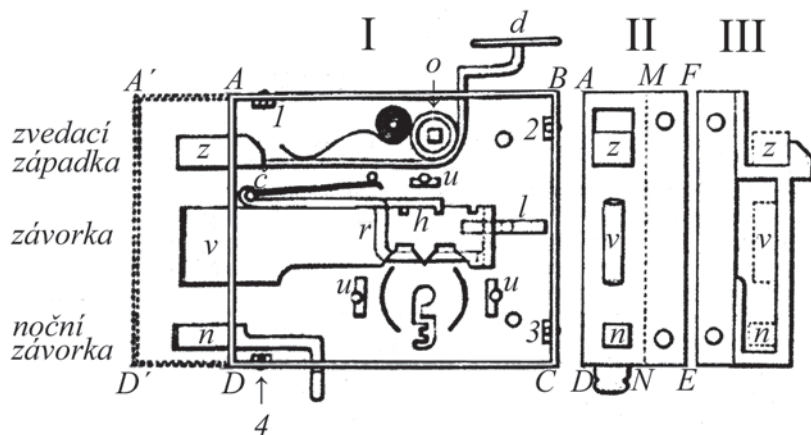
Obr. 48: Skříňový (dnes krabicový) zámek se zvedací západkou (Kastenschloss mit hebender Falle, n., f.).
