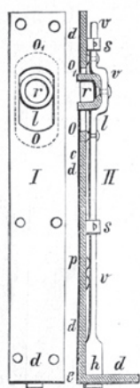
Obr. 35: Náprstková zástrčka v nejběžnější literatuře (převzato z A. O. F. Večeř, o. c. v pozn. 12, s. 38, obr. 89).
