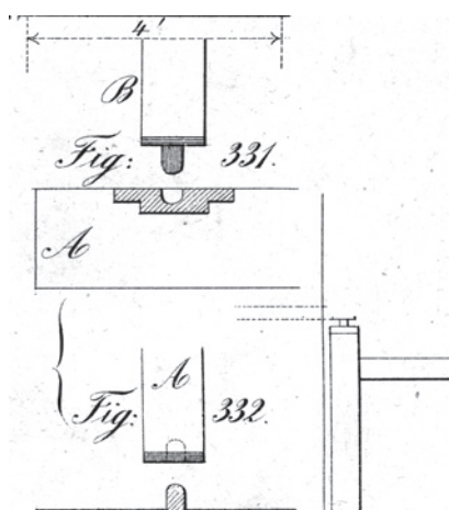
Obr. 19: Čep a pánev uvádí Joendl, který upřednostňoval pánev nahoře s ohledem na zanášení (převzato z J. P. Joendl, o. c. v pozn. 11. tab. 12, č. 331–333).
