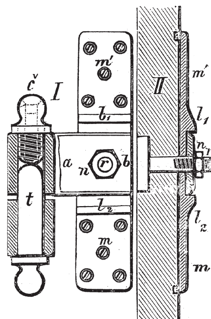
Obr. 6: Střední pásy byly velmi často minimalizovány: a – vlevo, okenní a dveřní křížový závěs (převzato z T. Hölzel, o. c. v pozn. 3, tab. 43, 44); b – upravo, pevný dveřní závěs (převzato z A. O. F. Večeř, o. c. v pozn. 12, s. 30, obr. 58).
