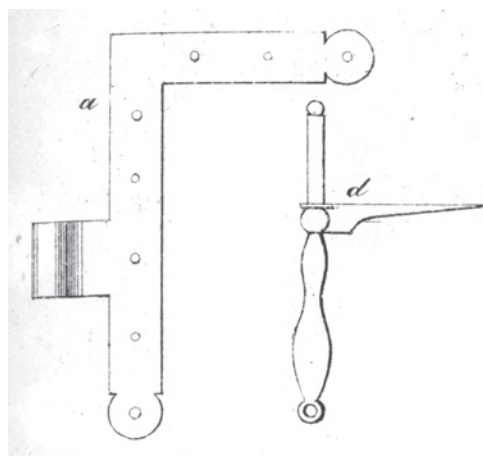
Obr. 9: Okenní a dveřní kování v Renwersově vzorníku z roku 1794: a – úhlové závěsy ve variantě s opěradlem a bez opěradla (HKA Wien, Kommerz Böhmen); b – jednodušší okenní úhlový závěs a závěsník s opěradlem u Hölzela, který úhlový závěs nadále považoval za standard, ač zapuštěné závěsy (viz níže) byly již dávno známy (převzato z T. Hölzel, o. c. v pozn. 3, tab. 44).
