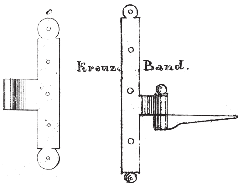
Obr. 6: Střední pásy byly velmi často minimalizovány: a – vlevo, okenní a dveřní křížový závěs (převzato z T. Hölzel, o. c. v pozn. 3, tab. 43, 44); b – upravo, pevný dveřní závěs (převzato z A. O. F. Večeř, o. c. v pozn. 12, s. 30, obr. 58).
