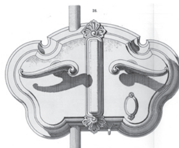
Obr. 60–64: Dalším krokem k estetickému pojednání zámku byly změny, kde obě části – vlastní zámek i celé ústrojí bývajícího zapadacího plechu – byly stejně široké. Tyto zámky existují od baroku, zná je Renwers (HKA Wien, Kommerz Böhmen) i Hölzel, který je nazývá vídeňský zámek (Wiener Schloss, n.) (převzato z T. Hölzel, o. c. v pozn. 3, tab. 6, 7, 18). J. Storck a kol. k roku 1876 uvádí funkčně podobný jako „starý francouzský zámek“ (vpravo), ač připouští, že tyto zámky se vyskytují ve Vídni, Francii, Anglii i Itálii (převzato z J. Storck – G. Gugitz – F. Paulik, o. c. v pozn. 10, sv. 2., tab. 12).
