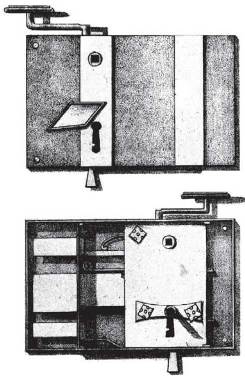
Obr. 53: Vnitřní mechanismus zámku (zde u krytých zámků, které jsou ve variantě se západkou, závorkou i noční závorkou). Velká část zámků neměla noční závorku, řada zámků měla pouze mechanismus západky, část zámků dle potřeby pouze mechanismus závorky. Západka (Falle, f.) – zvedací západka (hebende Falle, f.), zvaná německá. Mohla být pouze u zámků nezapuštěných.
