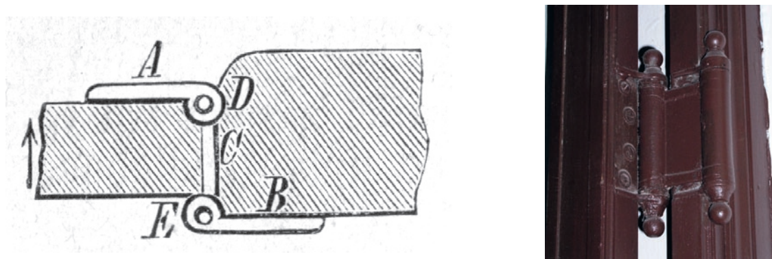
Obr. 23: a – střední závěs (převzato z A. O. F. Večeř, o. c. v pozn. 12, s. 32, obr. 63); b – kyvné dveře na téže principu, Praha – Hlavní nádraží (foto J. Škabradla).
