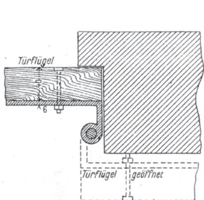
Obr. 18: Závěs lomený či odnášecí – různé varianty, nastupují však ve větším měřítku až na přelomu 19. a 20. století: a – vlevo dle Titschera 17) (převzato z F. Titscher, o. c. v pozn. 17. tab. 60); b – uprostřed závěs na okenici výkladce, aby se vyhnul bosáží, Libochovice (okres Litoměřice); c – vpravo závěs u interiérových skleněných dveří ze začátku 20. století v Desfourském paláci v Praze.
