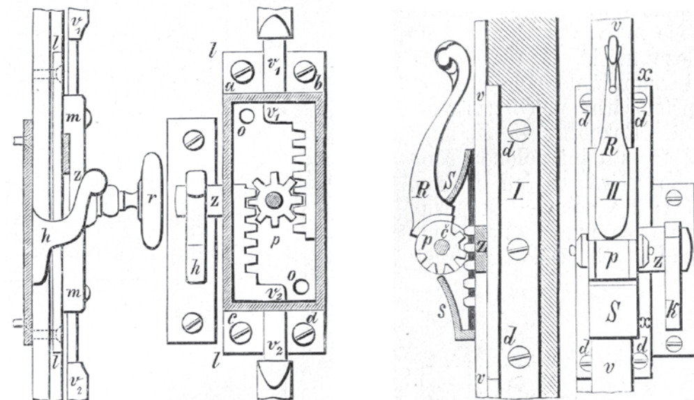
Obr. 42: Ve vypracované a nejpřehlednější podobě má hřebenový baskulík opět Večeřovo dílo: a – základem byl samozřejmě baskulík se dvěma tyčemi a dvěma hřebeny; b – méně byla používána varianta s jednou tyčí a jedním hřebem. Na Večeřových vyobrazeních je součástí zavírání druhého křídla navíc zapuštěný obrtlík (převzato z A. O. F. Večeř, o. c. v pozn. 12, s. 39–40, obr. 91, 92).
