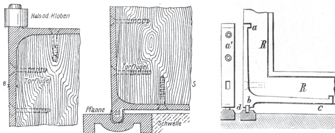
Obr. 21: Čepový závěs: a – pro těžká vrata v Titscherově práci, nahoře držel čep krček, dole pánev (převzato z F. Titscher, o. c. v pozn. 17, tab. 60, č. 6); b – pro pokojové dveře byly využívány skrytější systémy čepů či kolíků (převzato z A. O. F. Večeř, o. c. v pozn. 12, s. 31, obr. 59, 60).
