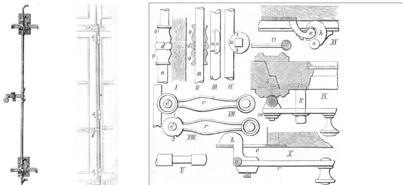
Obr. 37: Españolety jsou uváděny prakticky ve všech zámečnických dílech počínaje Duhamelem; a – zde v kombinaci s dalším zavíracím mechanismem (převzato z H-L. Duhamel du Monceau, o. c. v pozn. 4, tab. 15, obr. 18); b, c – nejpřehlednější jsou zakresleny u Večeře, kdy byl systém již několika generacemi vylepšován, aby hák nahoře a dole okno dotahoval (převzato z A. O. F. Večeř, o. c. v pozn. 12, s. 40-41, obr. 95-96).
