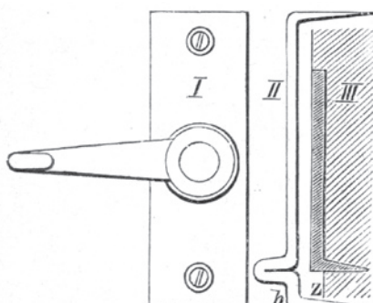
Obr. 24: a – vlevo: Večeř má nejucelenější přehled obrtlíků určených pro zavírání jednoho křídla okna od nejjednodušších připevněných vrutem či zanáťovanými do plechu; b – vpravo: v dokonalejších případech okenní lištu chránil drát či plíšek s ozubem (převzato z A. O. F. Večeř, o. c. v pozn. 12, s. 34–35, obr. 76 a 77).
