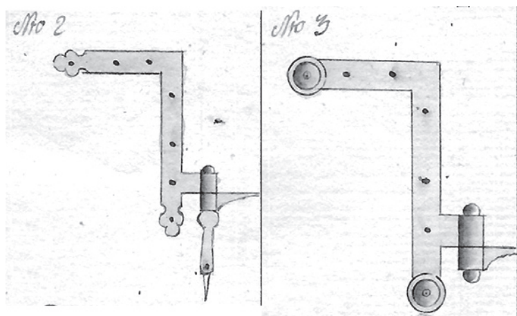
Obr. 9: Okenní a dveřní kování v Renwersově vzorníku z roku 1794: a – úhlové závěsy ve variantě s opěradlem a bez opěradla (HKA Wien, Kommerz Böhmen); b – jednodušší okenní úhlový závěs a závěsník s opěradlem u Hölzela, který úhlový závěs nadále považoval za standard, ač zapuštěné závěsy (viz níže) byly již dávno známy (převzato z T. Hölzel, o. c. v pozn. 3, tab. 44).
